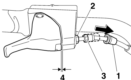
1 Copertura di gomma 2 Controdado 3 Registro 4 Gioco della leva dell'acceleratore
