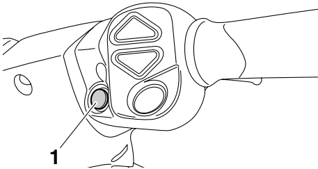
1 Interruttore "NO-WAKE MODE"
