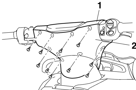
1 Copri-manubrio anteriore 2 Copri-manubrio posteriore
