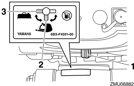
1. Rubinetto del carburante
