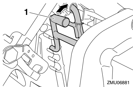
1. Barra di supporto tilt
