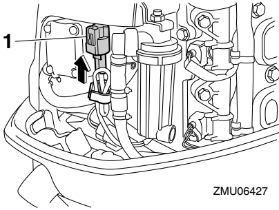
1. Accoppiatore dell'interruttore rilevamento acqua
