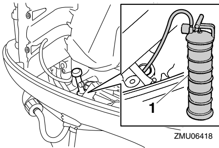
1. Estrattore
