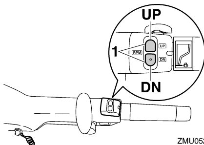
1. Interruttore di regime di traino variabile
