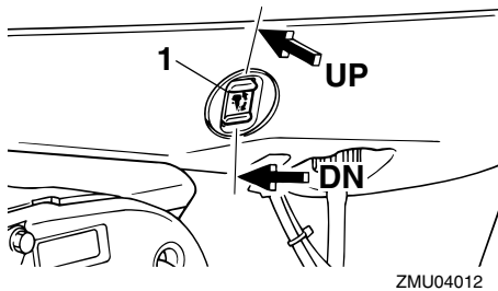
1. Interruttore PTT
