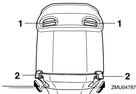
1. Griglia di aspirazione aria 2. Leva(e) di aggancio/sgancio calandra
