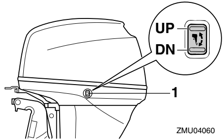
1. Interruttore PTT
