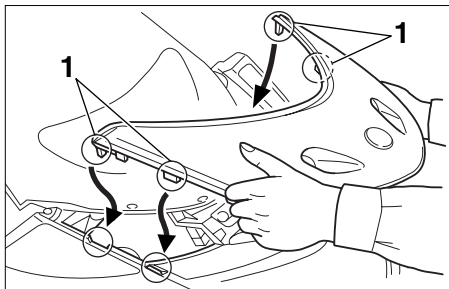
1. Linguette (x4)
