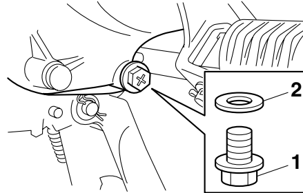
1. Getriebeöl-Ablassschraube 2. Dichtung
