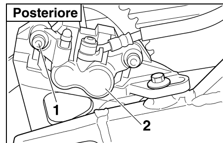
1. Bullone 2. Pinza freno posteriore
