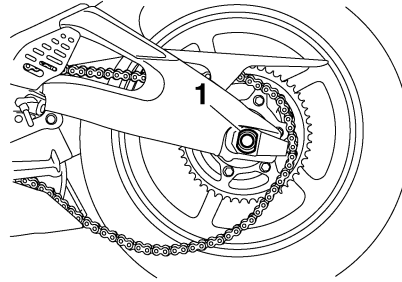
1. Perno ruota
