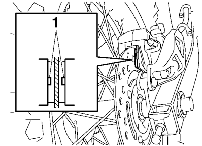
1. Verschleißanzeigergrille des Bremsbelags
