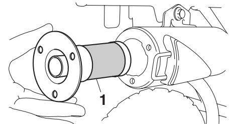
1. Funkenfänger
