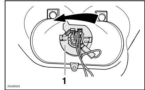
1. Gloeilamphouder
