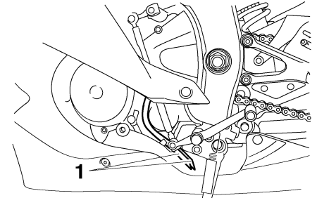
1. Tubetto di sfiato/troppo pieno del serbatoio carburante
