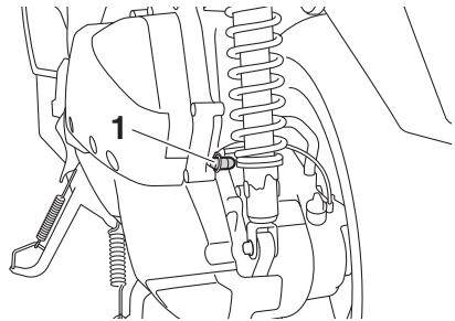
1. Tubo d'ispezione del filtro dell'aria
