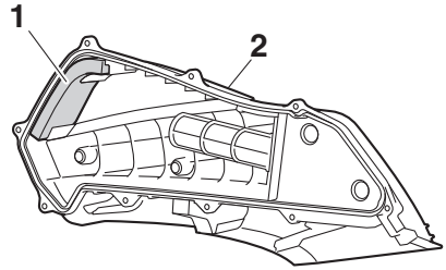
1. Elemento sub-filtrante 2. Coperchio della scatola del filtro dell'aria
