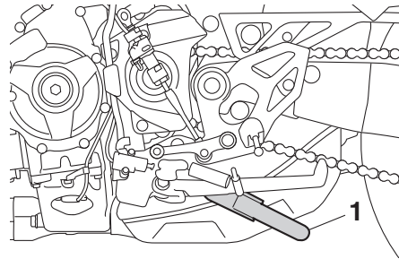
1. Barra stabilizzatrice
