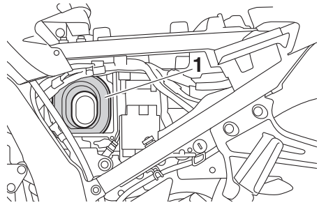
1. Elemento del filtro dell'aria
