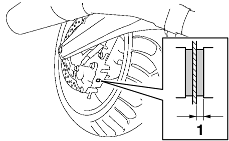
1. Spessore rivestimento pastiglia freno
