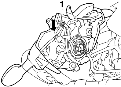
1. Connettore luce di posizione
