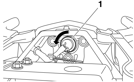
1. Cavetto portalampada fanalino posteriore/stop
