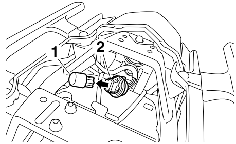
1. Lampada fanalino posteriore/stop 2. Cavetto portalampada fanalino posteriore/stop
