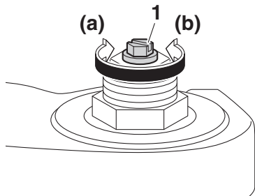
1. Vite di regolazione dello smorzamento in estensione
