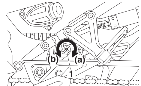
1. Vite di regolazione dello smorzamento in estensione
