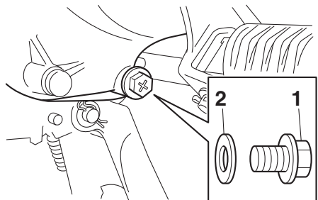
1. Getriebeöl-Ablassschraube 2. Dichtung
