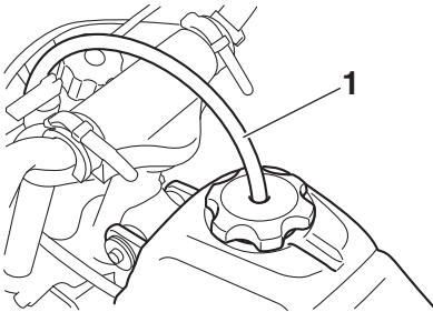
1. Kraftstofftank-Belüftungsschlauch
