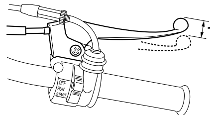
1. Garde du levier de frein avant
