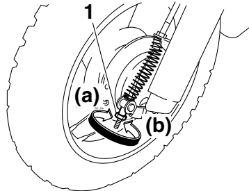
1. Einstellmutter für das Spiel des Handbremshebels
