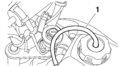
1. Kraftstofftank-Belüftungsschlauch
