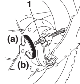
1. Einstellmutter für das Spiel des Fußbremshebels
