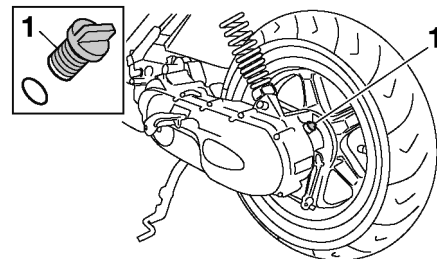
1. Tappo del bocchettone riempimento olio trasmissione finale
