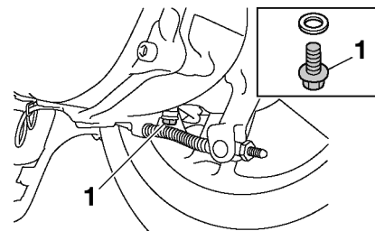
1. Bullone di drenaggio olio trasmissione finale
